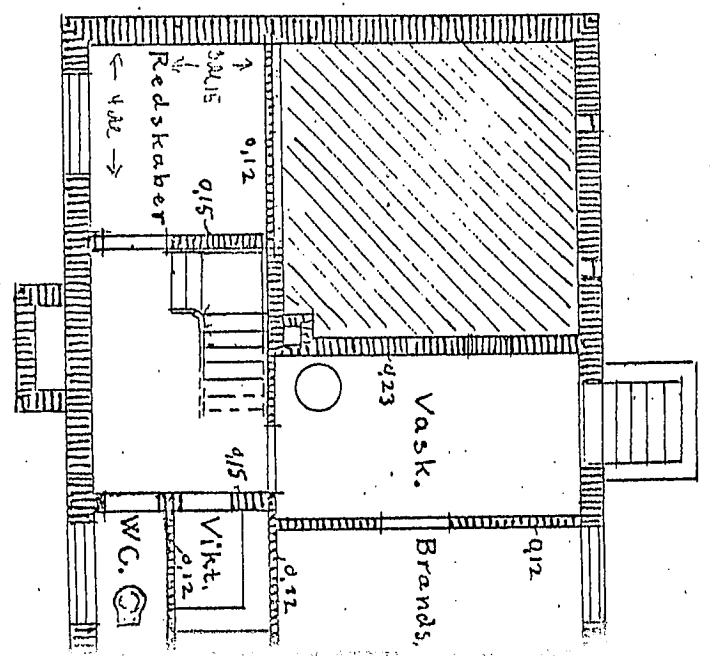
Hus D. Kælderplan
