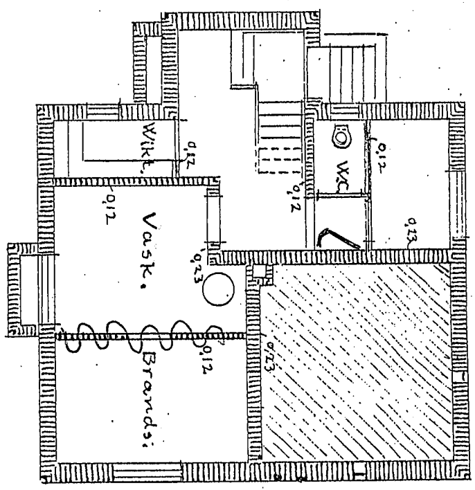
Hus C. Kælderplan.
